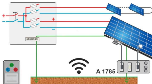
Figura 4-4: Misura di parametri ambientali (Collegamenti a MI 3114 o MI 3115)
