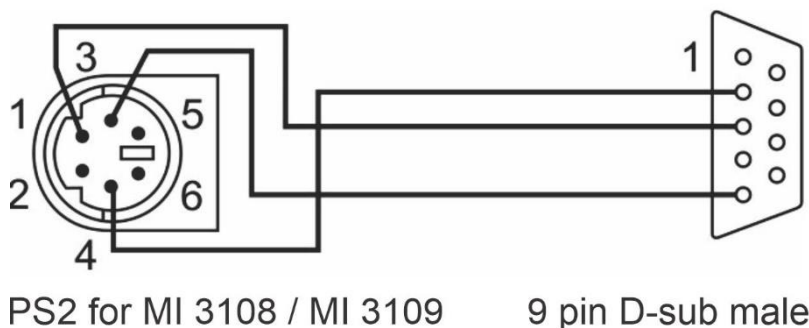
Figura 5-1: Collegamento di interfaccia per l'adattatore per cavo da RS232 (maschio) a PS/2
