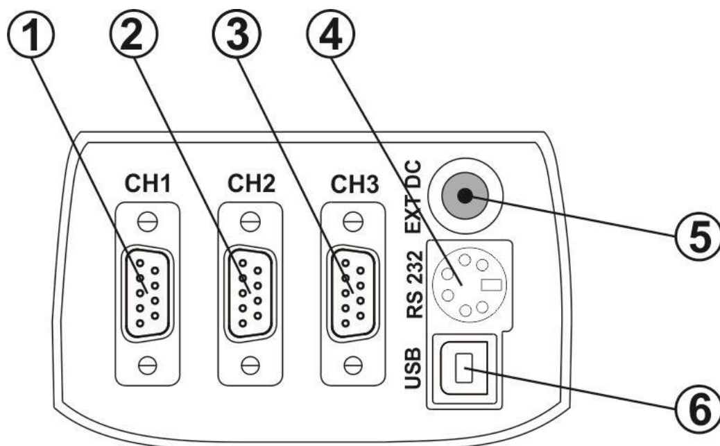
Figura 2-2: Pannello connettori
