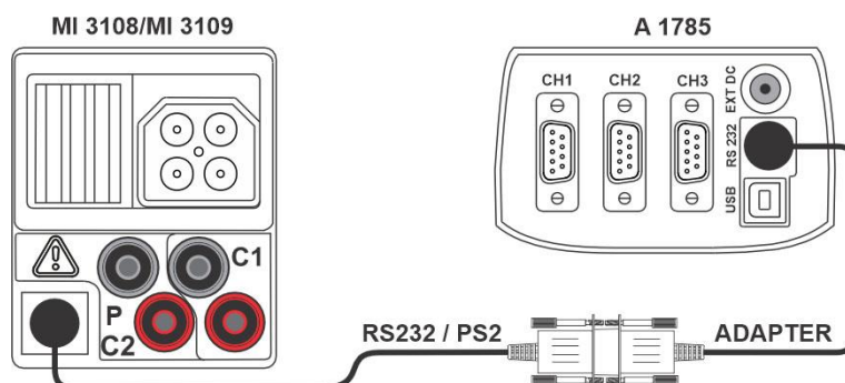
Figura 5-2 Collegamento degli strumenti durante la sincronizzazione
