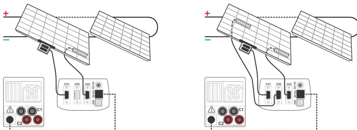
Figura 4-2: Misura di parametri ambientali (Collegamento di sonde)
