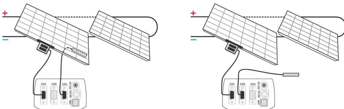
Figura 4-2: Misura di parametri ambientali (Collegamento di sonde)
